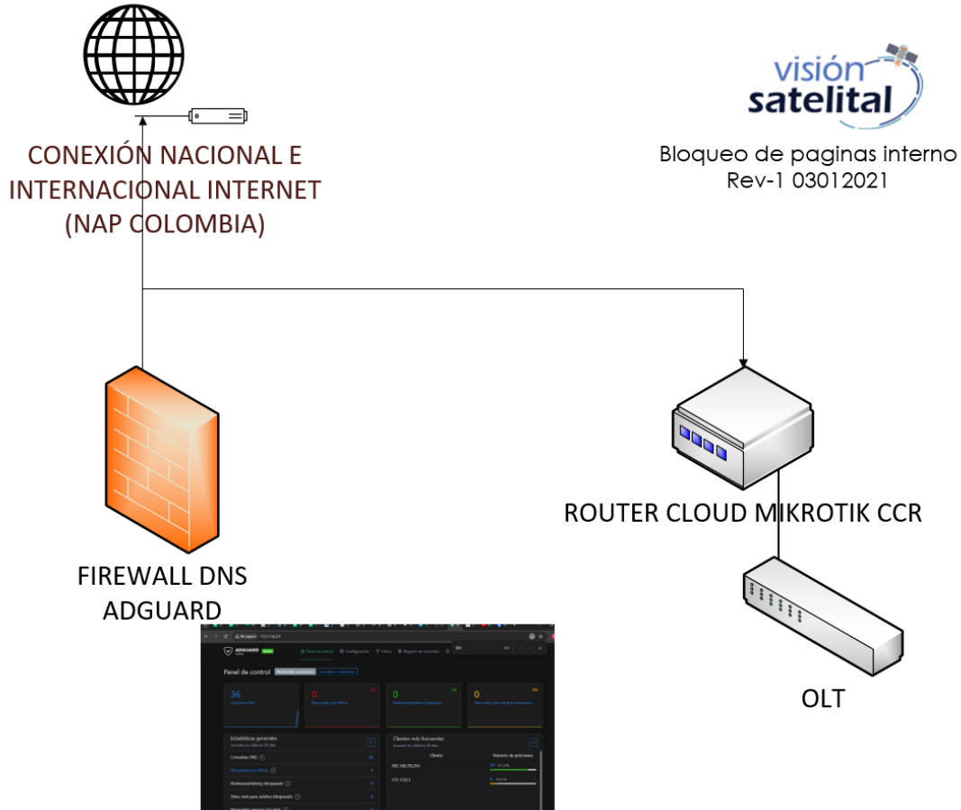
Diagrama básico
